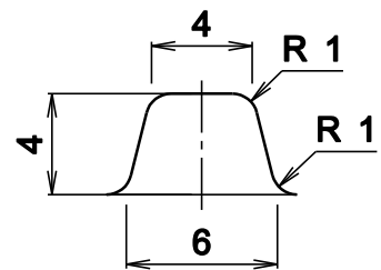
DETTAGLIO DELLA TACCA OPPOSTA AL LETTORE CAVITA' SCALA 3:1
